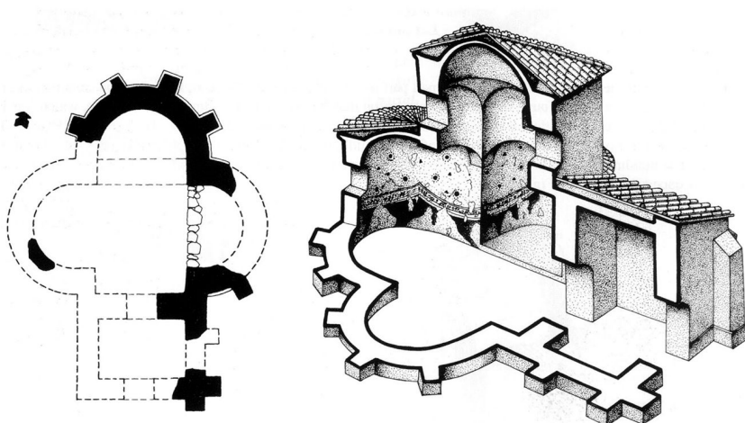
11 A pécsi cella trichora alaprajza az 1955-ben előkerült támpillérek kiegészítve és „robbantott” axonometrikus képe a megtalált falfestmények bemutatásával
