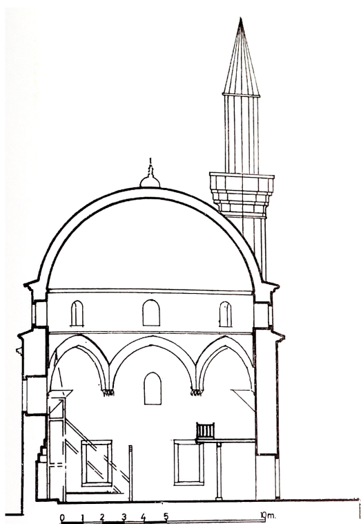
04 Bajrakli (Hüsszein Kethüda) Dzsámi, Belgrád, metszet és alaprajz
