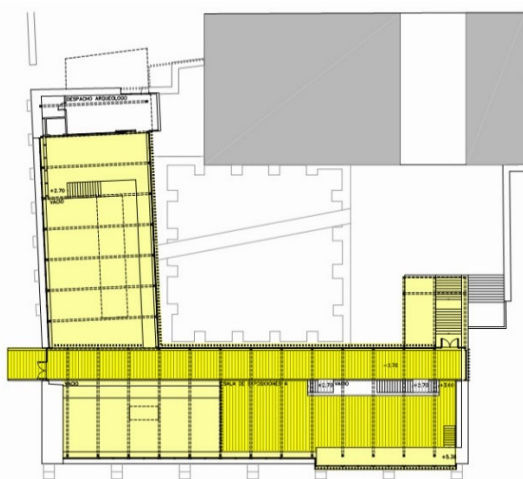
19. kép. Canvas Arquitectos: Várostörténeti Múzeum, Salamanca, Spanyolország, 2006. Forrás: ARQa
