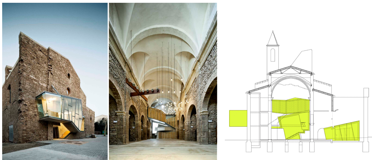
15. kép. David Closes: Sant Francesc Előadóközpont, Santpedor, Spanyolország, 2011. Forrás: Divisare
