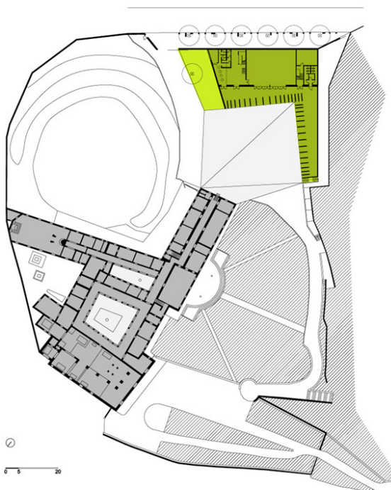
3. kép. Randić & Turato: II. János Pál fogadóépület, Rijeka, Horvátország, 2003-2008. Forrás: Archdaily
