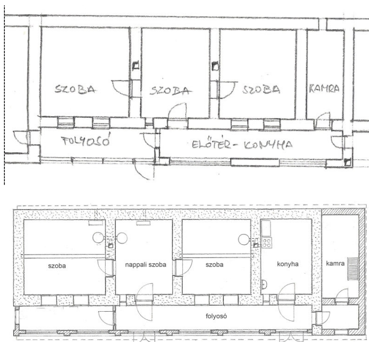
21. és 22. kép: Tornácbefalazás a Szeitz- és az Ignéczi-házban (saját ábra)
