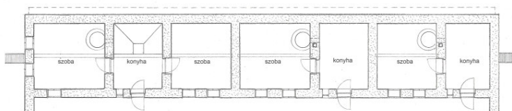
5. kép: Az Ignéczi-ház építéskori alaprajza (saját ábra)
