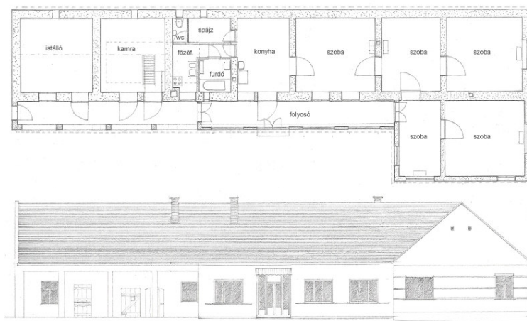
26. és 27. kép: A Bohner-ház alaprajza és udvari homlokzata az 1968-as átépítést követően (saját ábra)
