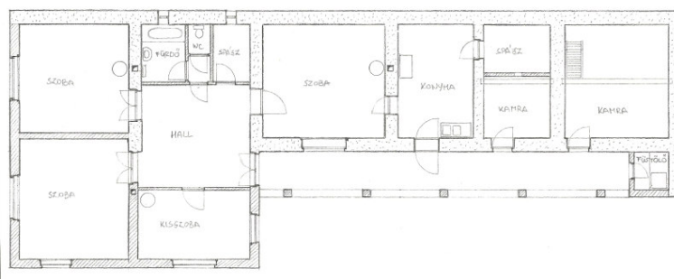
28. kép: A Huber-ház alaprajza az 1973-as átépítést követően (saját ábra)
