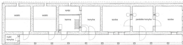
13. kép: Az Bohner-ház építéskori alaprajza a parádés konyhával (saját ábra)
