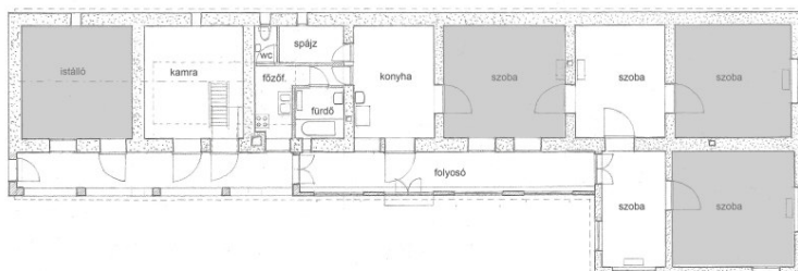
35. kép: Megüresedett helyiségek a Bohner-házban (saját ábra)
