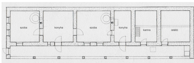
4. kép: A Huber-ház építéskori alaprajza (saját ábra)
