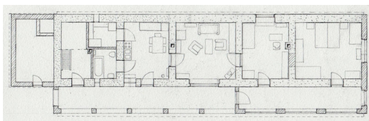
37. kép: A Mayer-ház alaprajza a 2000-es években, a nappalival (saját ábra)
