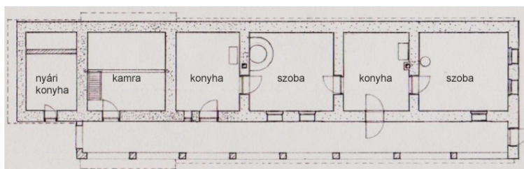
11. kép: A Mayer-ház alaprajza az 50-es években (saját ábra)
